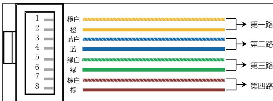
图 2.2-1 RJ45 线序
