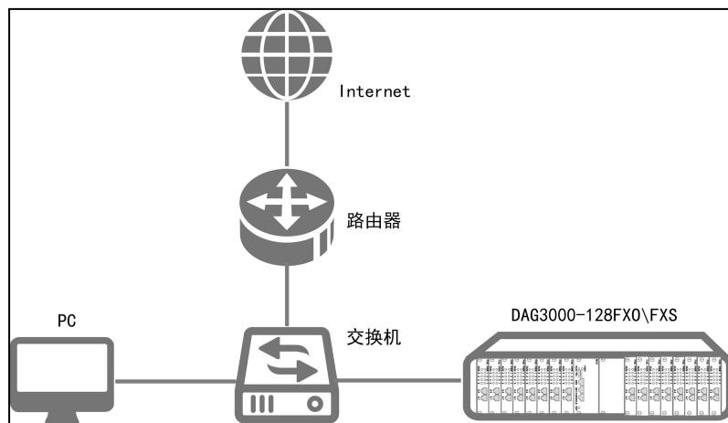
图 4.1-1 典型网络拓扑连接图
