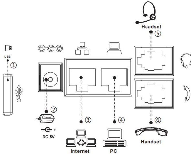
图 3 - 设备连接
