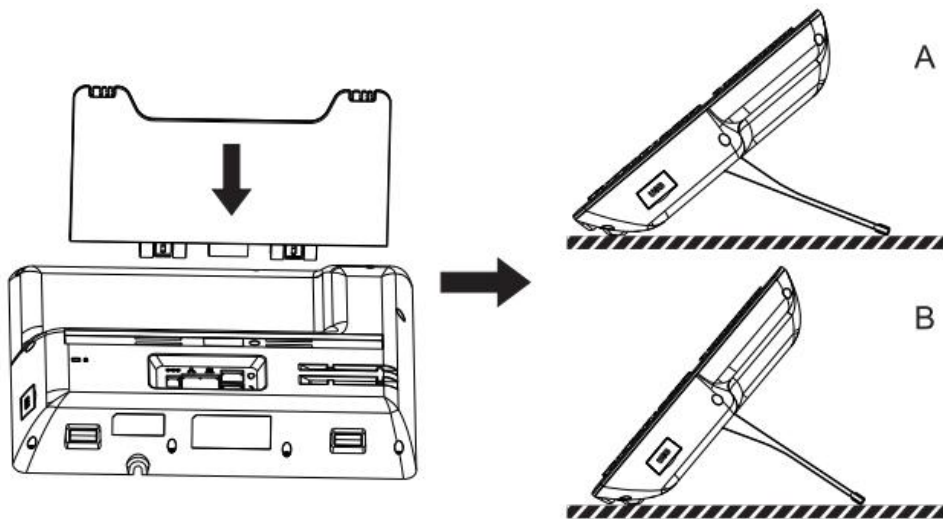
图 1 - 设备安装
