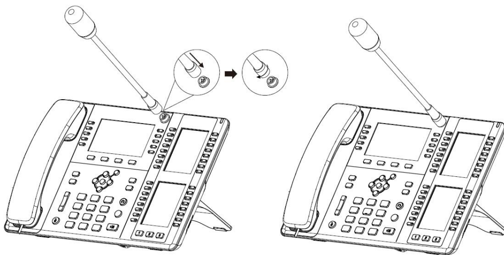
图 2 - 鹅颈麦克风安装(仅 X210i 支持)
