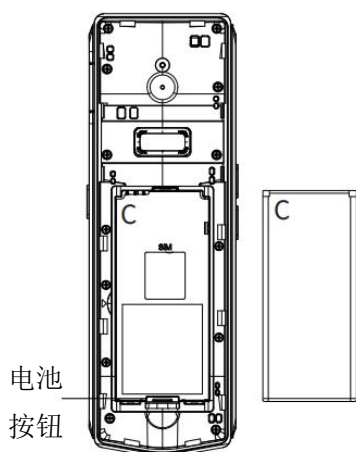
安装新电池
