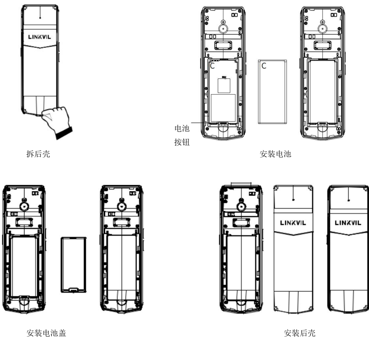
图 1- 安装电池
