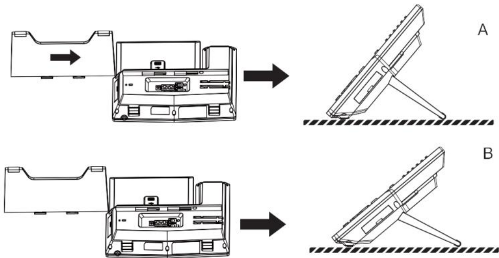
图 1- 桌面式话机安装
