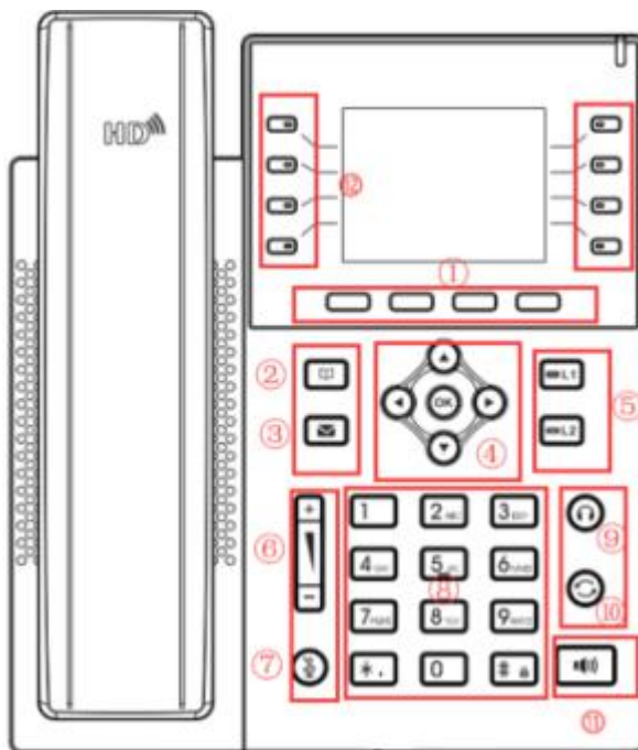
图 4 - 按键说明
