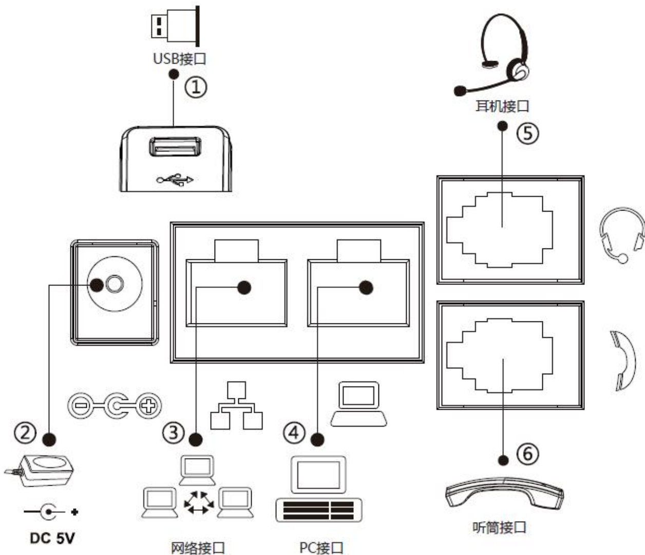
图 3 - 设备连接
