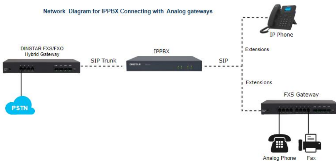
图1-6 应用拓扑图
